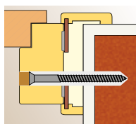
Szerelés téglafalba dübel és purhab segítségével
