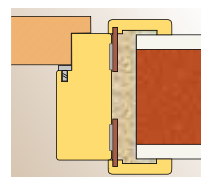
Szerelés téglafalba purhab segítségével.
