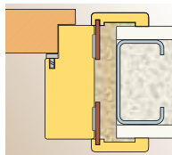
Szerelés gipszkarton falba purhab segítségével.
