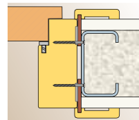
Szerelés gipszkarton falba csavarok segítségével.
